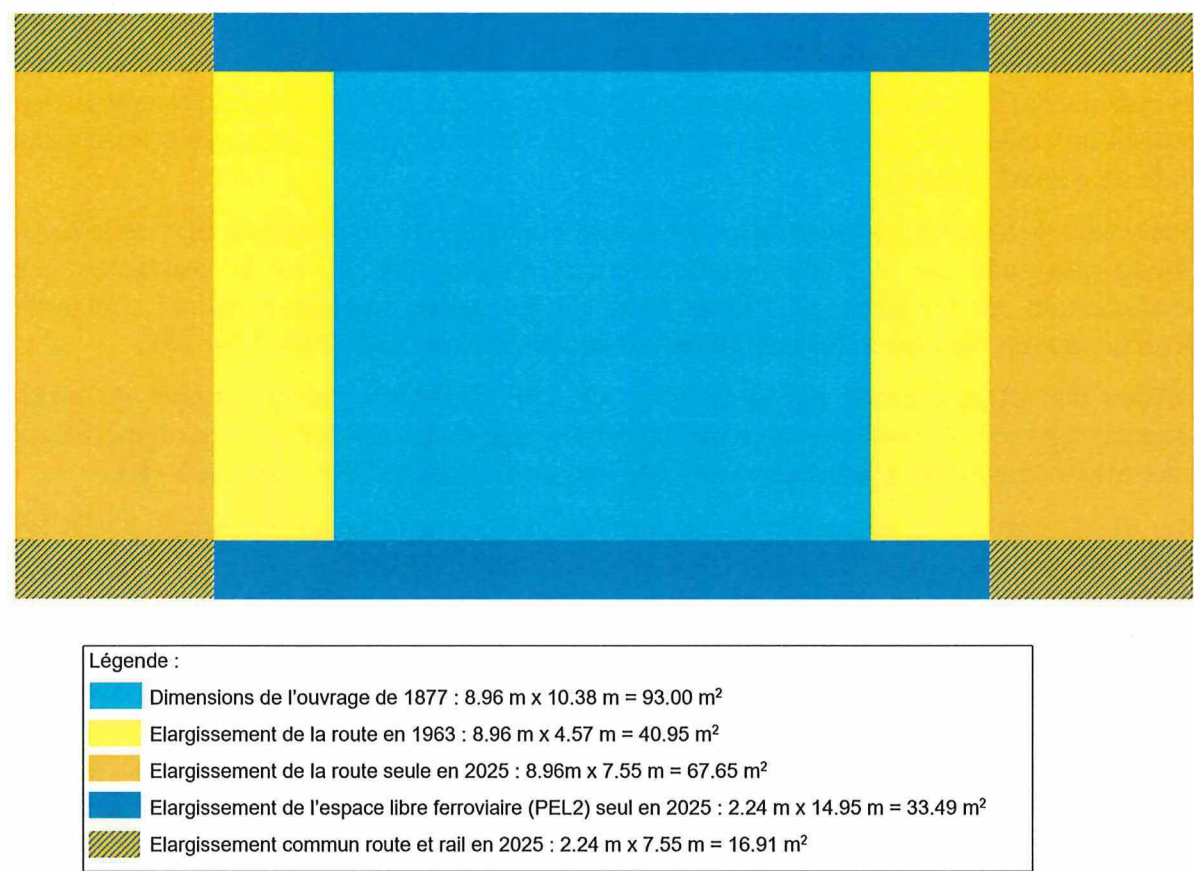
Figure 1 - Représentation schématique de l'évolution des dimensions de l'ouvrage
